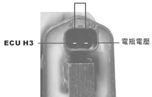
點火線圈一次迴路 0.5\Omega \sim 0.8\Omega 註： 0.63\Omega (23°C)
