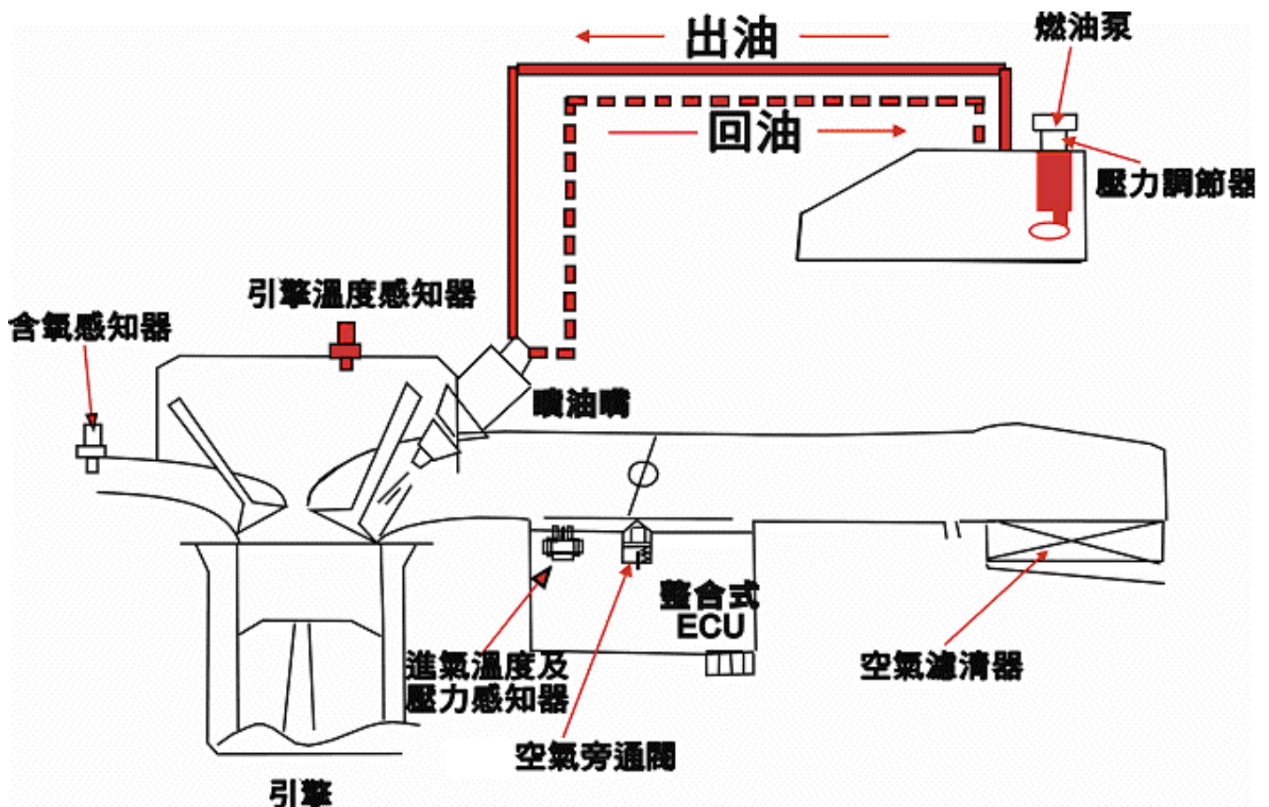
燃油噴射系統示意圖
