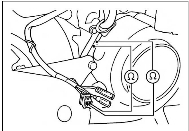
充電/照明線圈接頭
