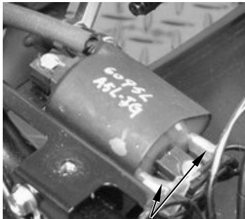
一次線圈端子電阻值量測
