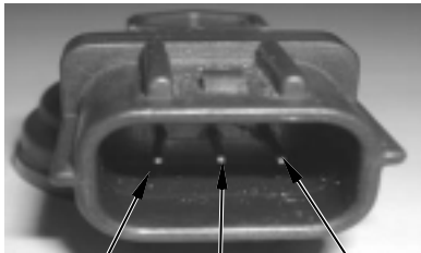
黃/黑 黑/紅 綠/紅
