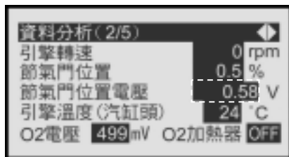
油門輸出訊號確認-全閉
