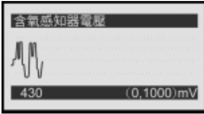
修正電壓數值變動的情形
