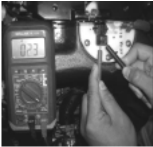
燃油泵電阻值量測
