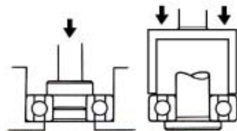
此兩種範例都會破壞軸承
