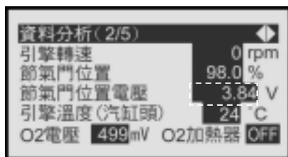
油門輸出訊號確認-全開
