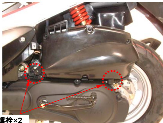
螺栓×2
