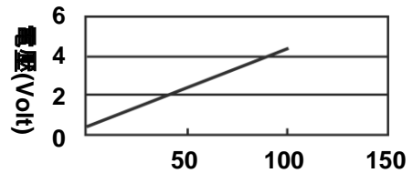
TPS 輸出電壓特性
