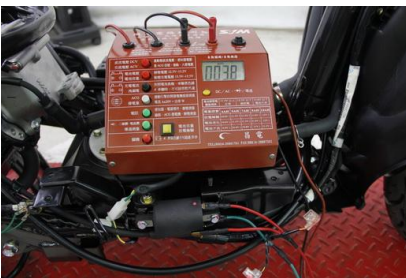
二次線圈端子電阻值量測
