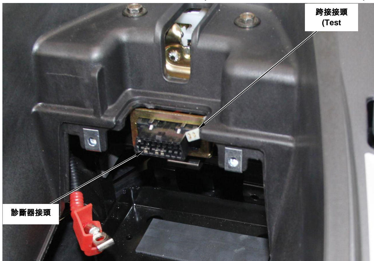
診斷器接頭與跨接接頭位置圖
