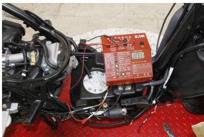
燃油泵電阻值量測
