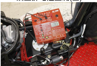
油量計電阻量測(滿)
